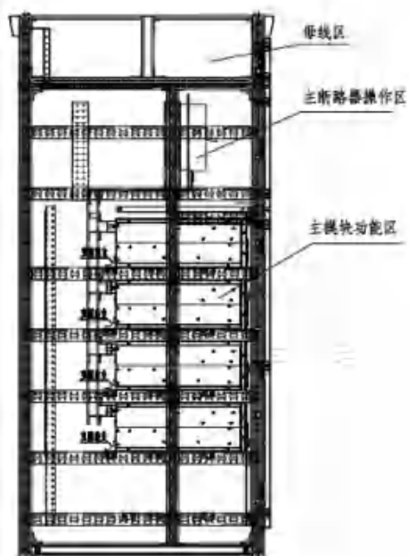
侧视
