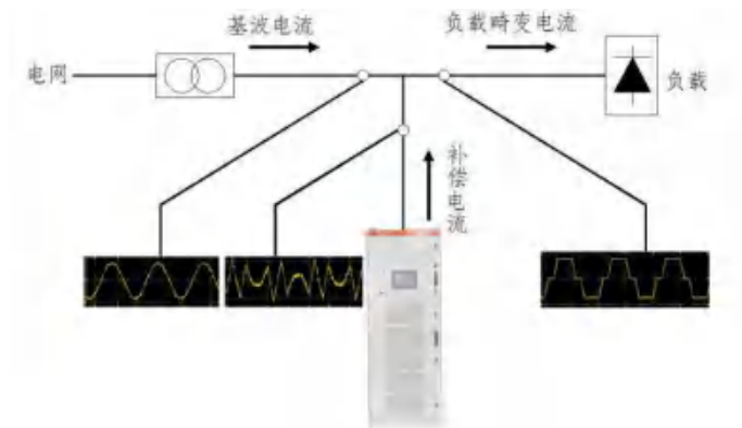
图3-1 AnSin 工作原理图
