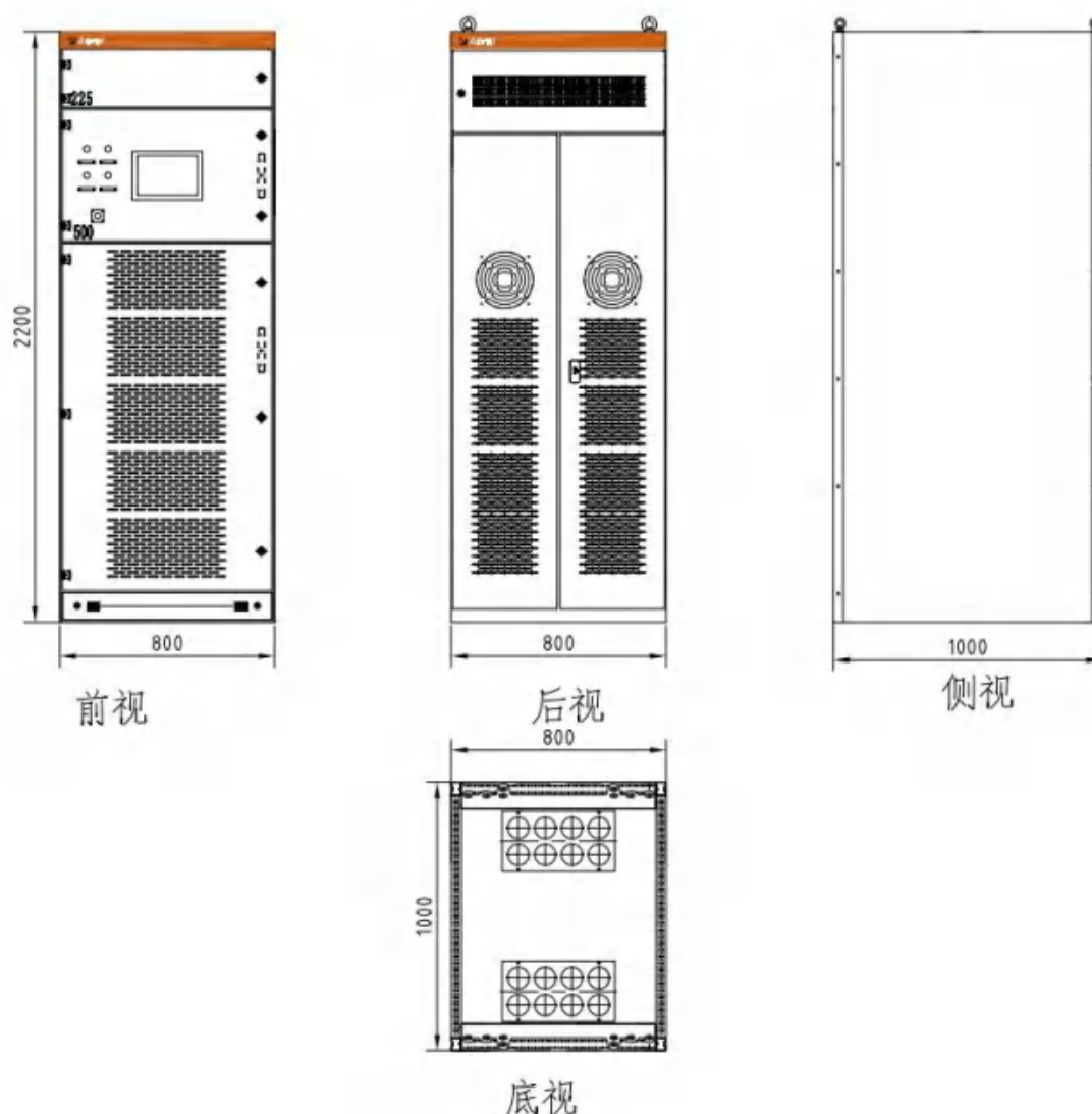
图4-4 600A整柜尺寸图
